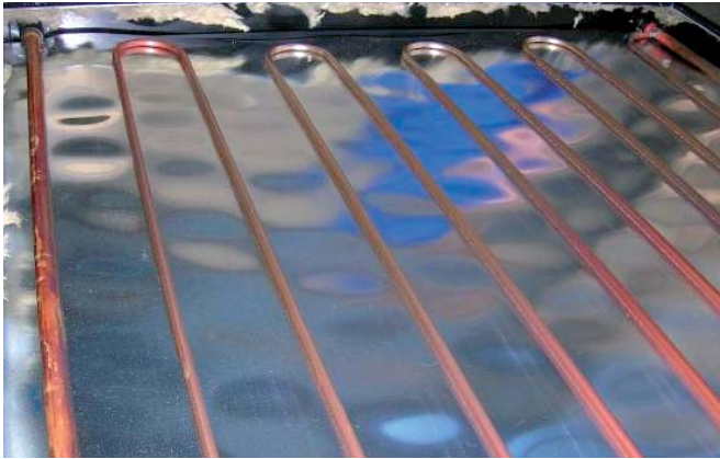
Bild 21: Verbindung Kupferrohre / Aluabsorber Picture 21: Connection copper tubes / alu absorber
