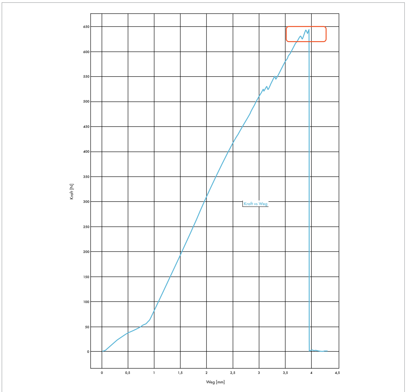
Abreißprobe Absorber Probe W
